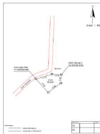
Gambar 13. Contoh Gambar Ukur Desa Langgini
