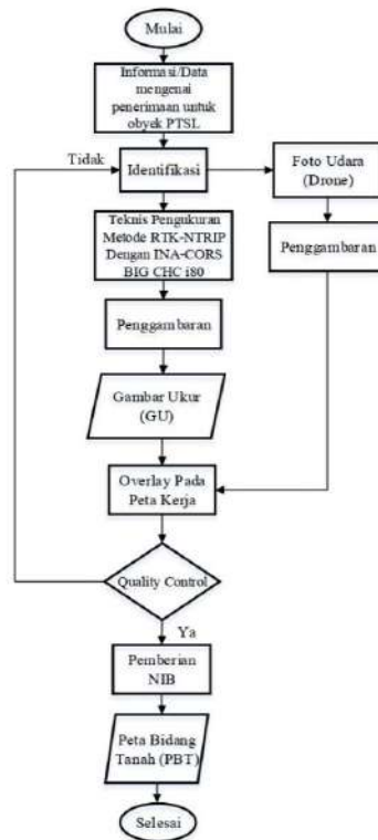
Gambar 2. Diagram Alir Pekerjaan
