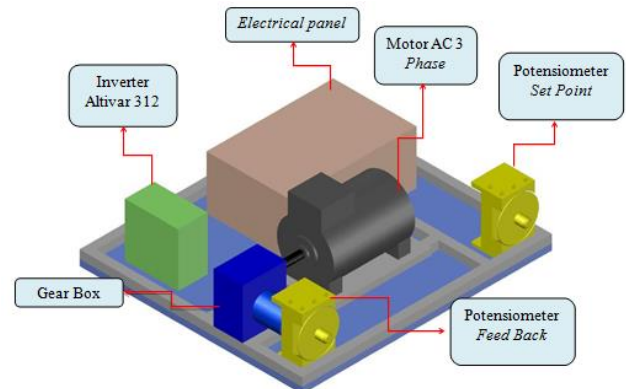
Gambar 3.2 Perancangan 3D
