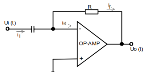
Gambar 2.4 Rangkaian Diferensiator
