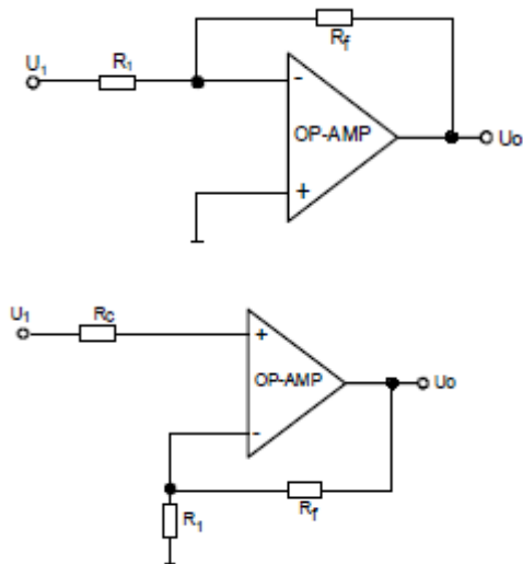
Gambar 2.2 Rangkaian OP-Amp
