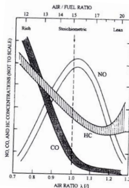
Gambar 2.2. Tipikal kurva ketiga polutan utama yang dihasilkan motor pembakaran dalam [6].
