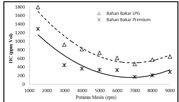
Gambar 4.3 Perbandingan kadar emisi hidrokarbon (HC) terhadap putaran mesin (rpm) pada kondisi full open throttle .
