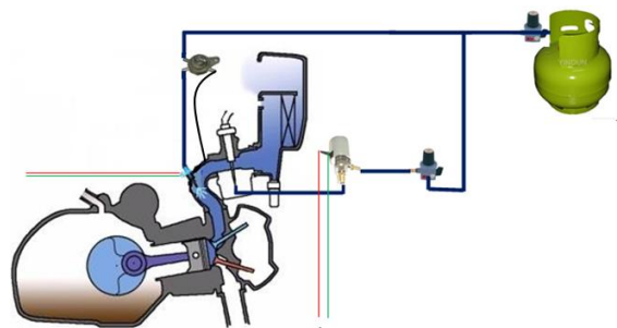
Gambar 3.2 Skema konverter kit
