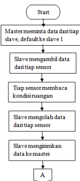
Gambar 3.2 Bagan Sistem Alat Node Slave
