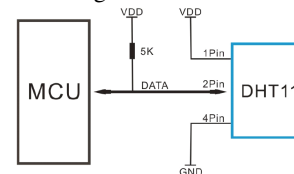
Gambar 2.3 Skema Rangkaian Sensor DHT11
