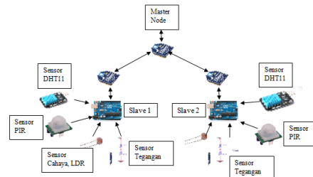
Gambar 3.2 Bagan Sistem Alat Node Slave
