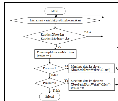
Gambar 3.13 Diagram Alir Form Home Komunikasi
