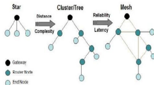
Gambar 2.1 Contoh Skema Topologi Star, Tree dan Mesh Pada Jaringan WSN
