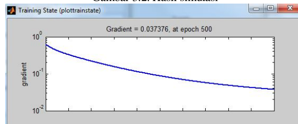
Gambar 3.2. Hasil simulasi
