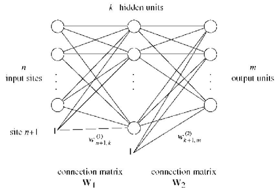
Gambar 2.1 Arsitektur Backpropagasi [5]
