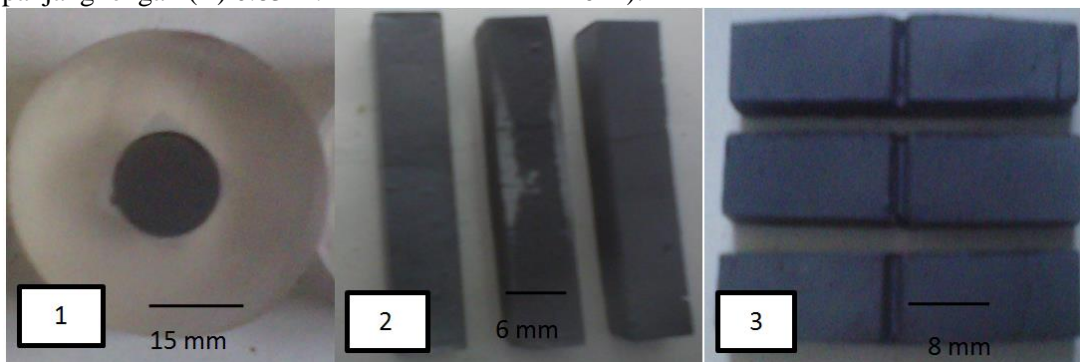
Gambar 4. Spesimen pengujian. 1) kekerasan 2) bending 3) impak
