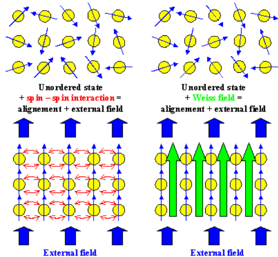
Gambar 1. Arah domain-domain dalam bahan ferromagnetic sebelum dan sesudah diberi medan magnet luar (Föll, 2004)
