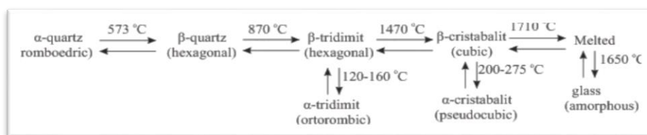
Gambar 3. Perubahan fase silika (Stefan dkk, 2011)
