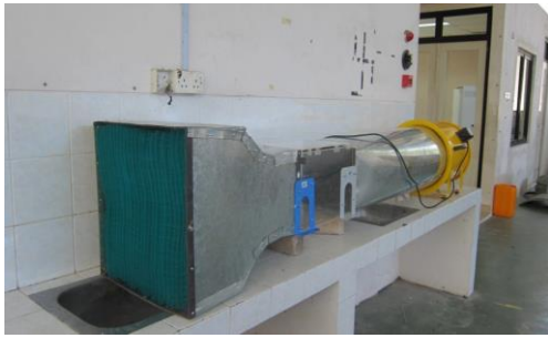
Gambar 3. Kerucut Kontraksi
