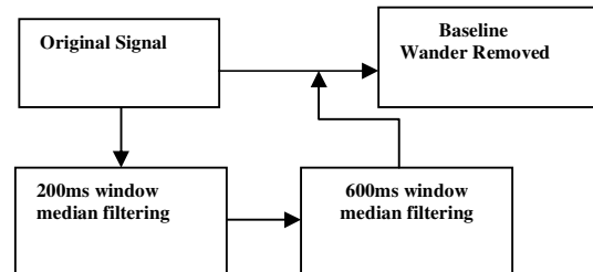
Gambar 2.1 Blok Diagram untuk Menghilangkan baseline wander
